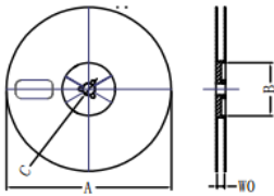
Reel Dimensions
