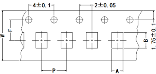
包装带尺寸图 Tape Size
