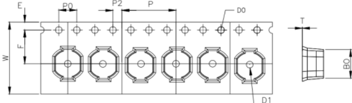
包装带尺寸图 Tape Size
