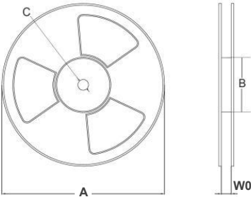
卷轴尺寸图 Reel Size
